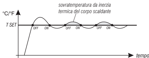
esempio tipo di regolazione proporzionale modulante
