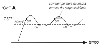
esempio tipo di regolazione differenziale
